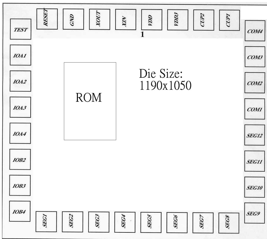
邦定图：（IC 底盘接地）
